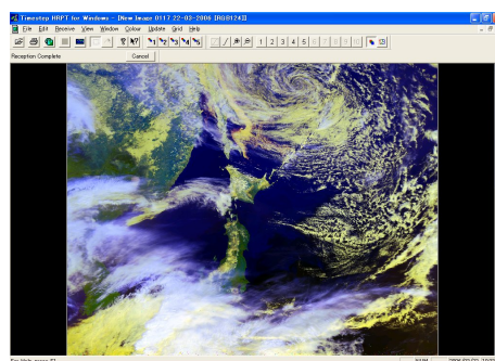
図 1.5 NOAA 衛星疑似カラー画像
