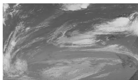
図 1.3 NOAA 衛星気象画像 (赤外波長域)
